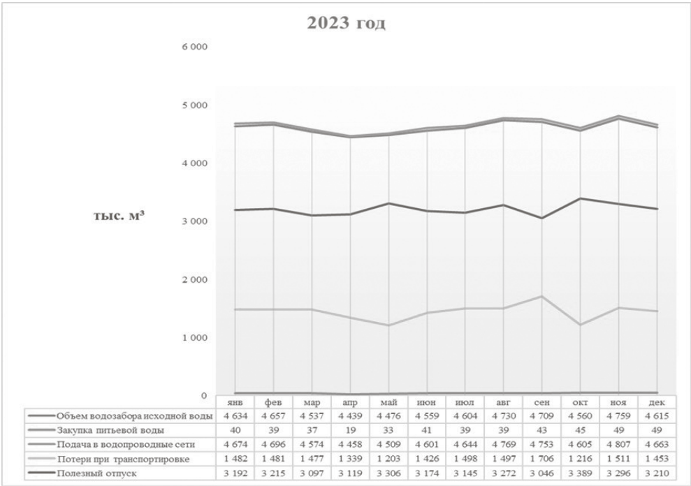
Рисунок 3.1 – Общий баланс подачи и реализации воды за 2023 год по ООО «РВК-Липецк»
