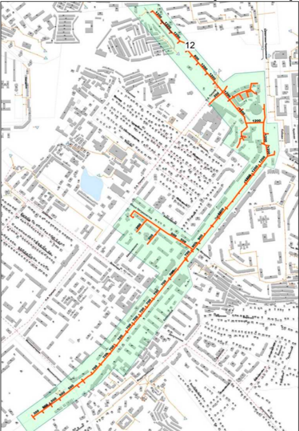
Рисунок 13 – Технологическая зона № 12 Технологическая зона № 13 Технологическая зона находится в микрорайонах № 4, 7. Сеть ливневой канализации проложена по ул. Космонавтов от дома № 20 до ул. Циолковского, по ул. Германа Титова от дома № 9/1 до ул. Космонавтов, по ул. Циолковского от дома № 3/1 до выпуска в Каменный Лог в районе гаражного кооператива «Мехземстрой». Общая протяженность сети технологической зоны № 13, согласно данным электронной модели, составляет 5 193 м. Диаметр трубопроводов различный от 150 до 900 мм. Площадь территории, покрываемой сетями технологической зоной № 13 составляет 64,07 Га. Технологическая зона представлена на рисунке 13.
