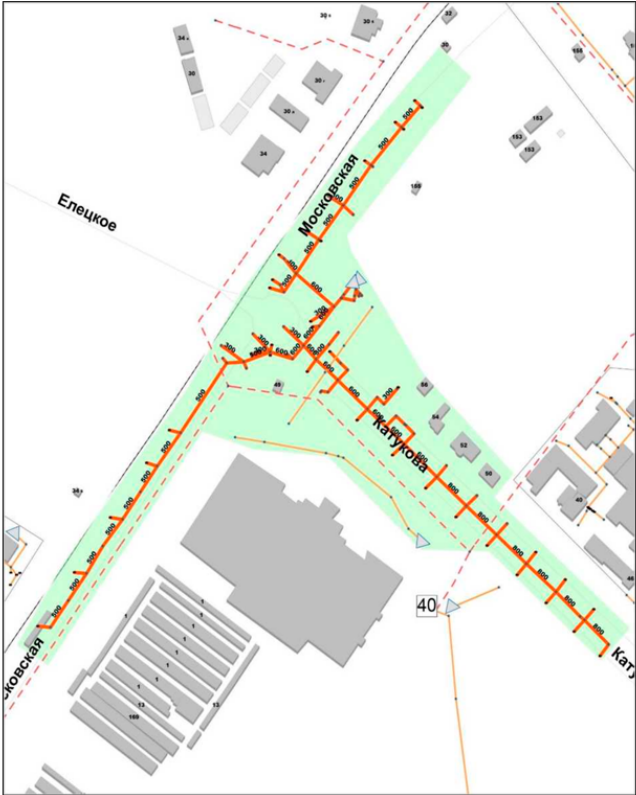
Рисунок 95 – Технологическая зона № 96 Технологическая зона № 97 Сеть ливневой канализации проложена в районе дома № 18а по ул. Юных натуралистов с последующим выпуском на очистные сооружения. Общая протяженность сети технологической зоны № 97 согласно данным электронной модели, составляет 134 м. Диаметр трубопроводов различный от 100 до 500 мм. Площадь территории, покрываемой сетями технологической зоной № 97 составляет 0,64 Га. Технологическая зона представлена на рисунке 95.
