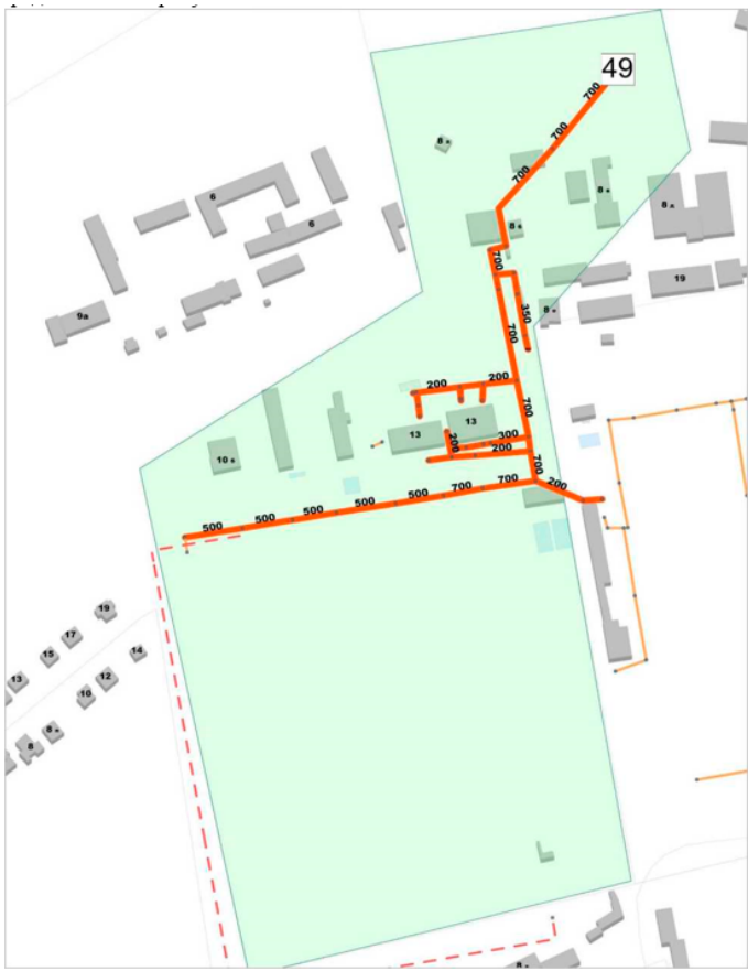
Рисунок 48 – Технологическая зона № 49 Технологическая зона № 50 Технологическая зона находится в районе «Опытной станции». Сеть ливневой канализации проложена на территории Тепличного комплекса в районе ул. Ботанической с выпуском в реку. Общая протяженность сети технологической зоны № 50, согласно данным электронной модели, составляет 2 300 м. Диаметр трубопроводов различный от 140 до 1200 мм. Площадь территории, покрываемой сетями технологической зоной № 50 составляет 45,78 Га. Технологическая зона представлена на рисунке 48.
