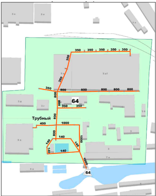
Рисунок 63 – Технологическая зона № 64 Технологическая зона № 65 Сеть ливневой канализации проложена на территории промплощадки в районе Трубно-го завода с последующим выпуском на рельеф далее самотёков в пруд. Общая протяженность сети технологической зоны № 65, согласно данным электронной модели, составляет 820 м. Диаметр трубопроводов различный от 150 до 600 мм. Площадь территории, покрываемой сетями технологической зоной № 65 составляет 3,08 Га. Технологическая зона представлена на рисунке 63.
