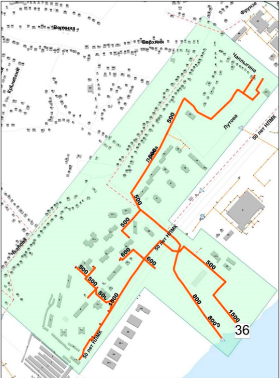
Рисунок 36 – Технологическая зона № 36 Технологическая зона № 37 Технологическая зона находится в микрорайоне № 15. Сеть ливневой канализации проложена по ул. Водопьянова от дома № 9 до дома № 29 с последующим выпуском в Каменный Лог. Общая протяженность сети технологической зоны № 37, согласно данным электронной модели, составляет 2 976 м. Диаметр трубопроводов различный от 150 до 1200 мм. Площадь территории, покрываемой сетями технологической зоной № 37 составляет 27,13 Га. Технологическая зона представлена на рисунке 36.
