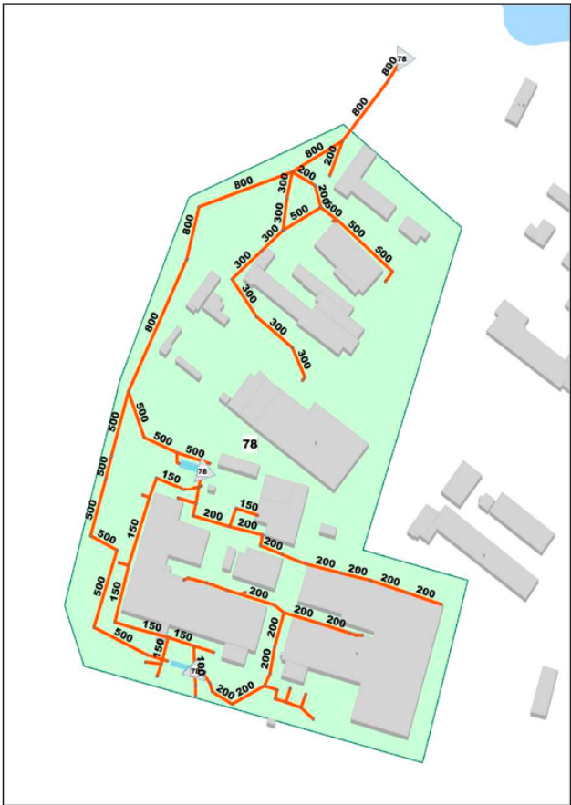
Рисунок 77 – Технологическая зона № 78 Технологическая зона № 79 Сеть ливневой канализации проложена на территории Липецкого Metallургического комбината «НЛМК». Общая протяженность сети технологической зоны № 79, согласно данным электронной модели, составляет 1 873 м. Диаметр трубопроводов различный от 200 до 900 мм. Площадь территории, покрываемой сетями технологической зоной № 79 составляет 11,03 Га. Технологическая зона представлена на рисунке 77.
