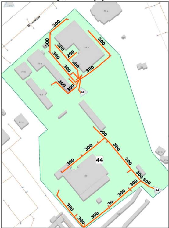
Рисунок 43 – Технологическая зона № 44 Технологическая зона № 45 Технологическая зона находится в районе Трубного завода. Сеть ливневой канализации проложена на территории трамвайного депо № 2 по ул. Полиграфической с выпуском в Каменный Лог в районе гаражного кооператива «Липчанин-6». Общая протяженность сети технологической зоны № 45, согласно данным электронной модели, составляет 1 966 м. Диаметр трубопроводов различный от 150 до 500 мм. Площадь территории, покрываемой сетями технологической зоной № 45 составляет 16,98 Га Технологическая зона представле- на на рисунке 43.
