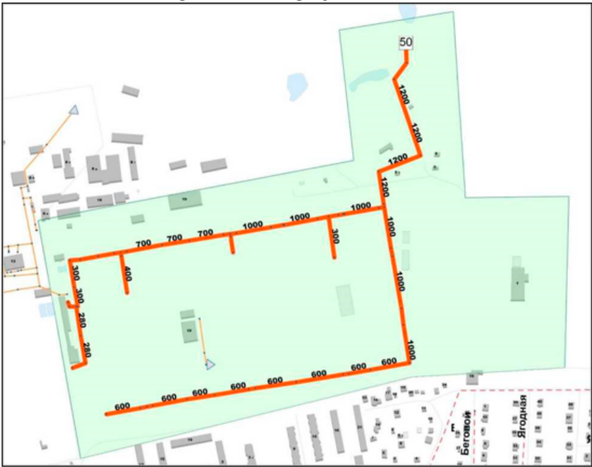
Рисунок 49 – Технологическая зона № 50 Технологическая зона № 51 Технологическая зона находится в микрорайоне «Новолипецк». Сеть ливневой канализации проложена по ул. Аносова от дома № 1 до дома № 20, по ул. Волжская от дома № 7 до дома № 11 по ул. береговой с выпуском в р. Воронеж за водной станцией в районе частного сектора. Общая протяженность сети технологической зоны № 51, согласно данным электронной модели, составляет 585 м. Диаметр трубопроводов различный от 300 до 900 мм. Площадь территории, покрываемой сетями технологической зоной № 51 составляет 10,96 Га. Технологическая зона представлена на рисунке 49.
