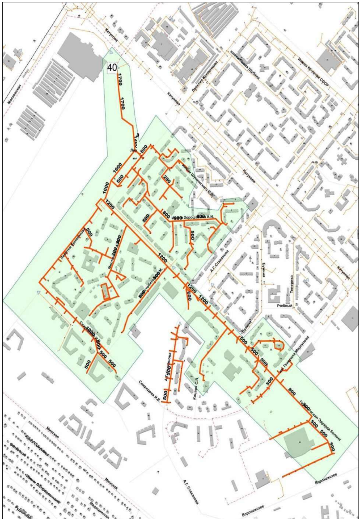
Рисунок 39 – Технологическая зона № 40
