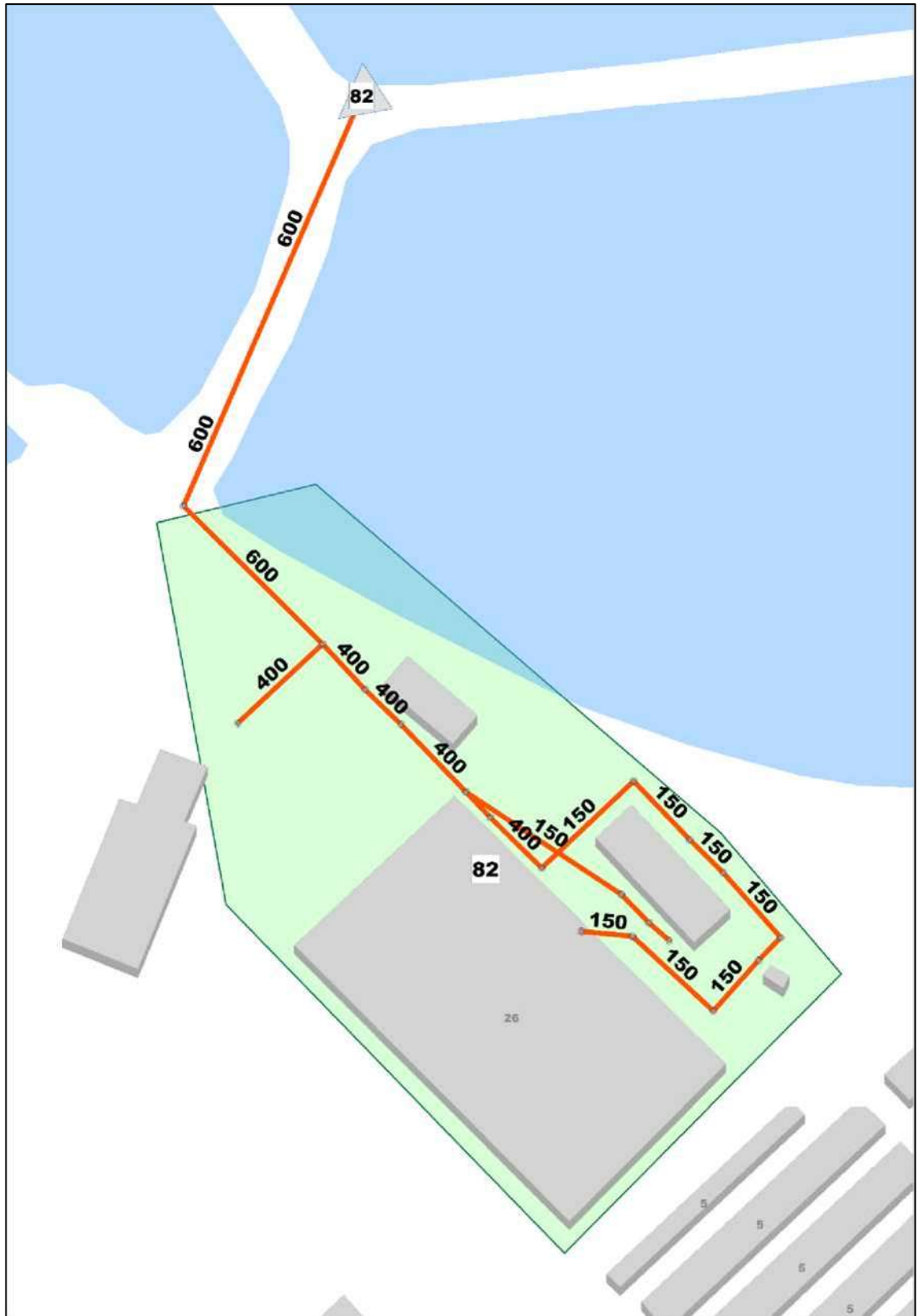
Рисунок 81 – Технологическая зона № 82
