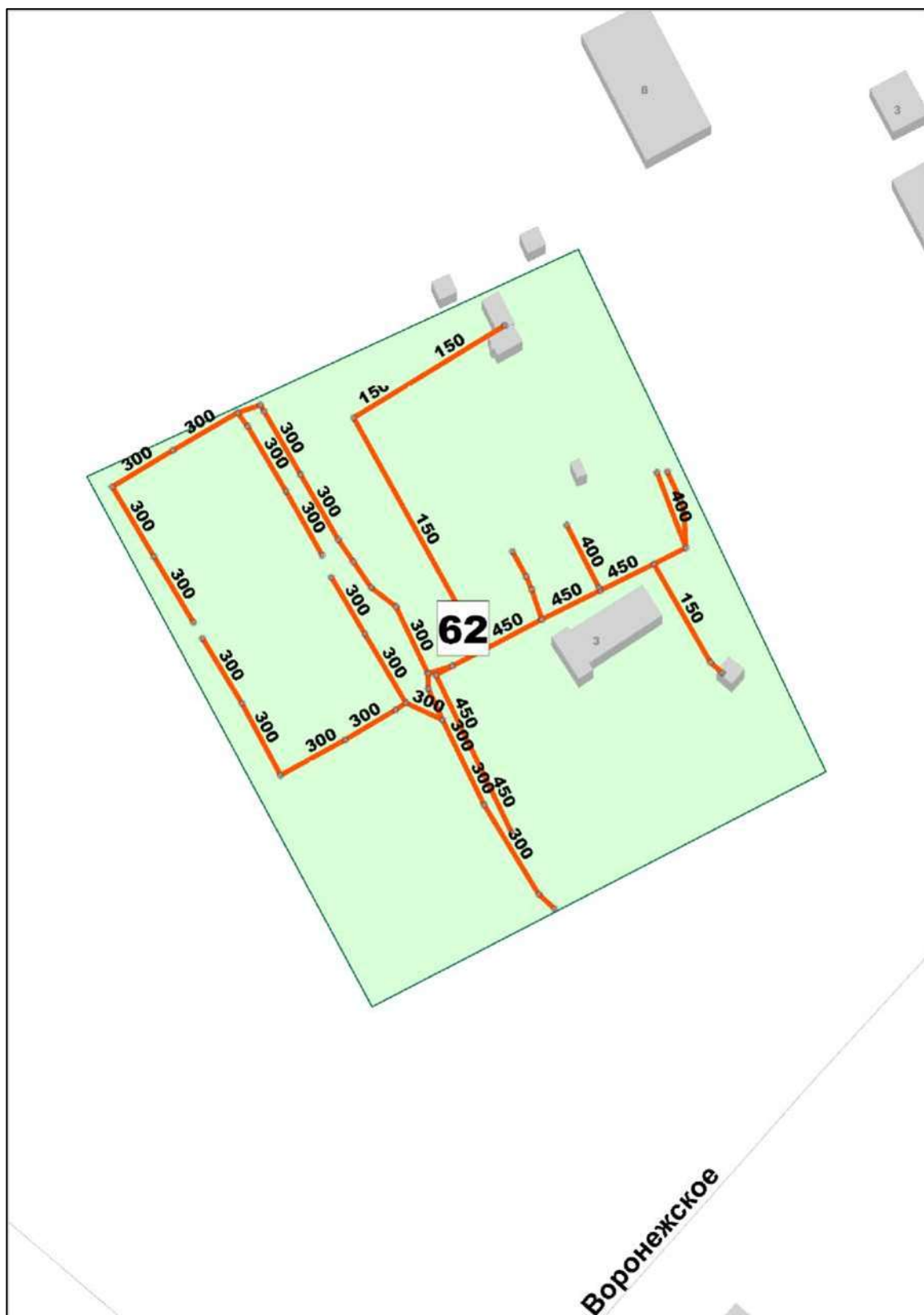
Рисунок 61 – Технологическая зона № 62
