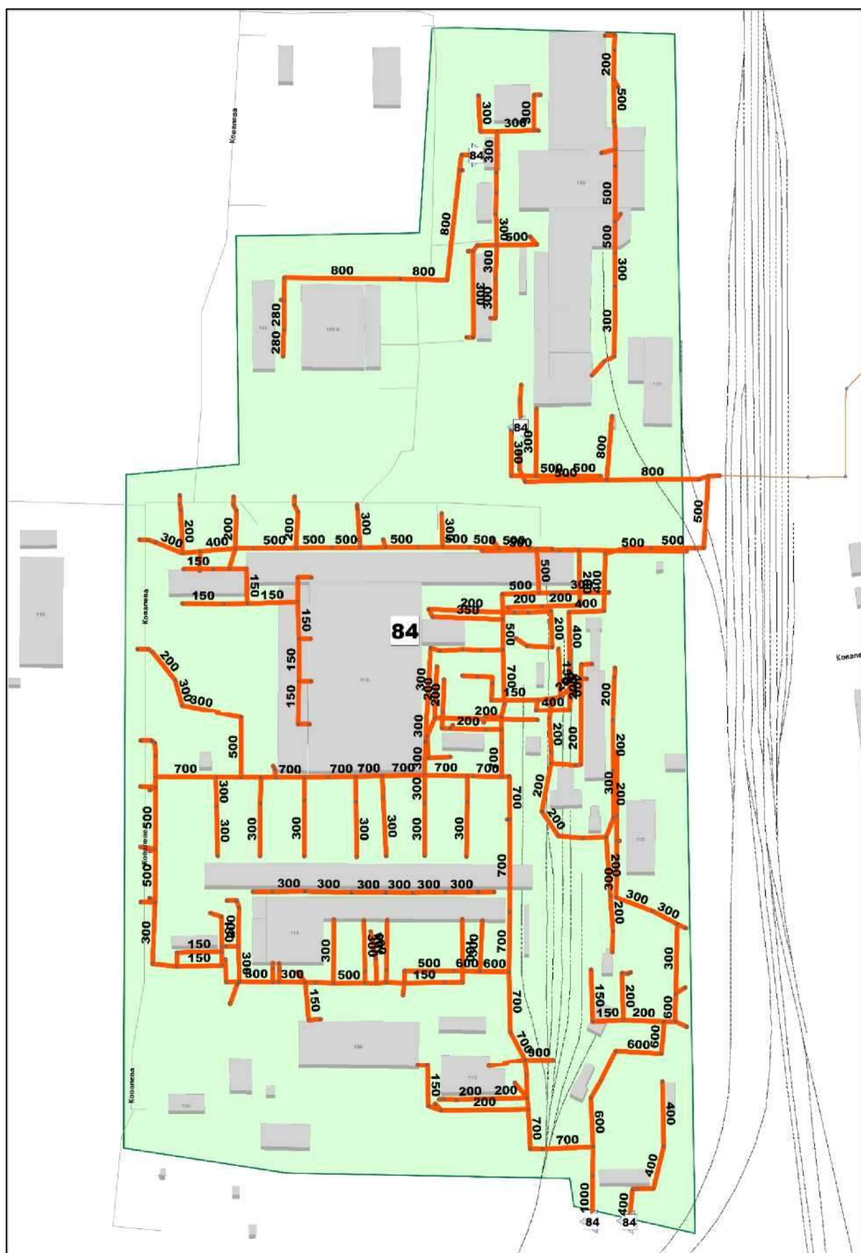
Рисунок 83 – Технологическая зона № 84
