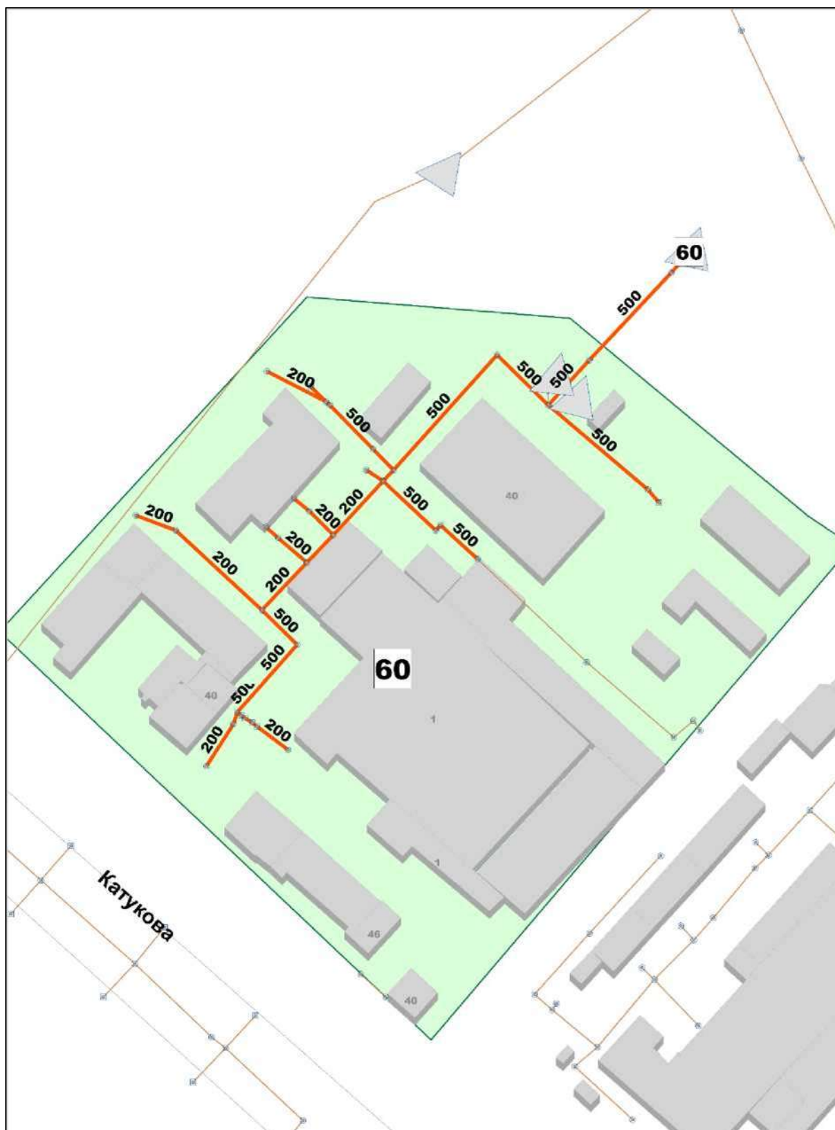
Рисунок 59 – Технологическая зона № 60
