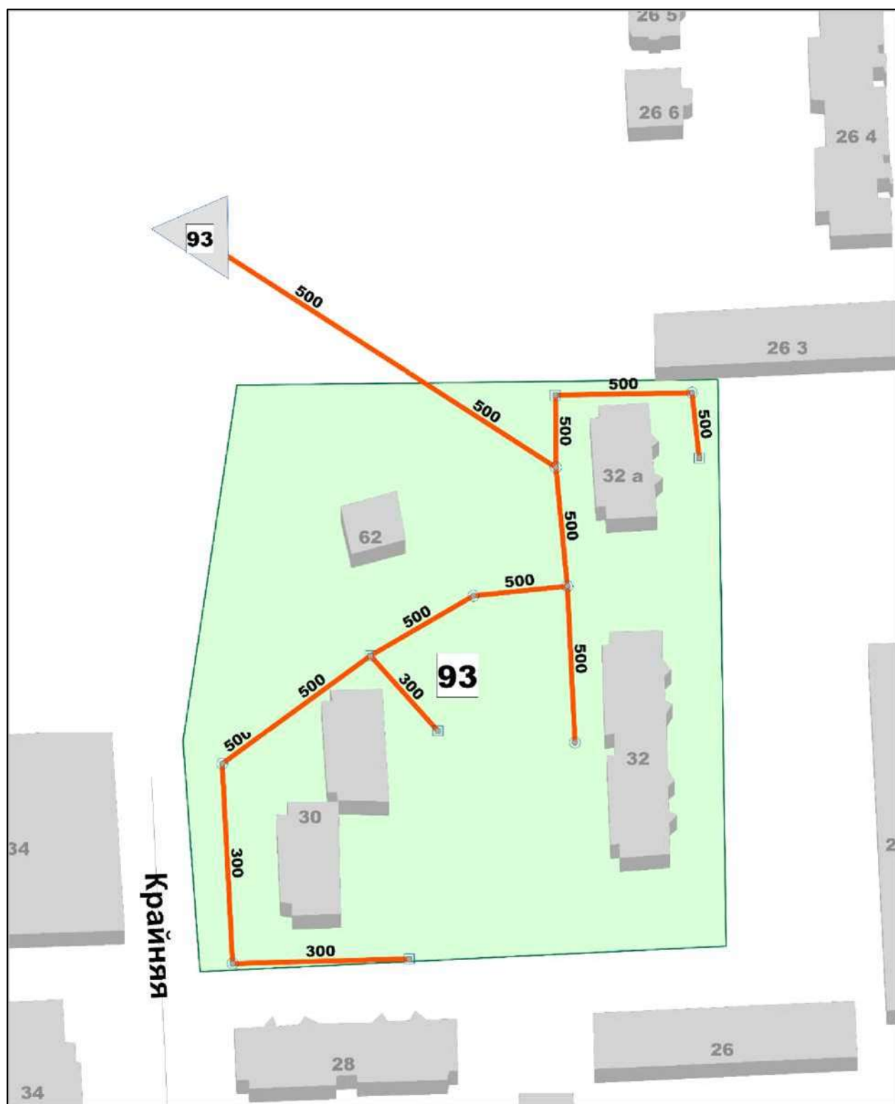
Рисунок 92 – Технологическая зона № 93
