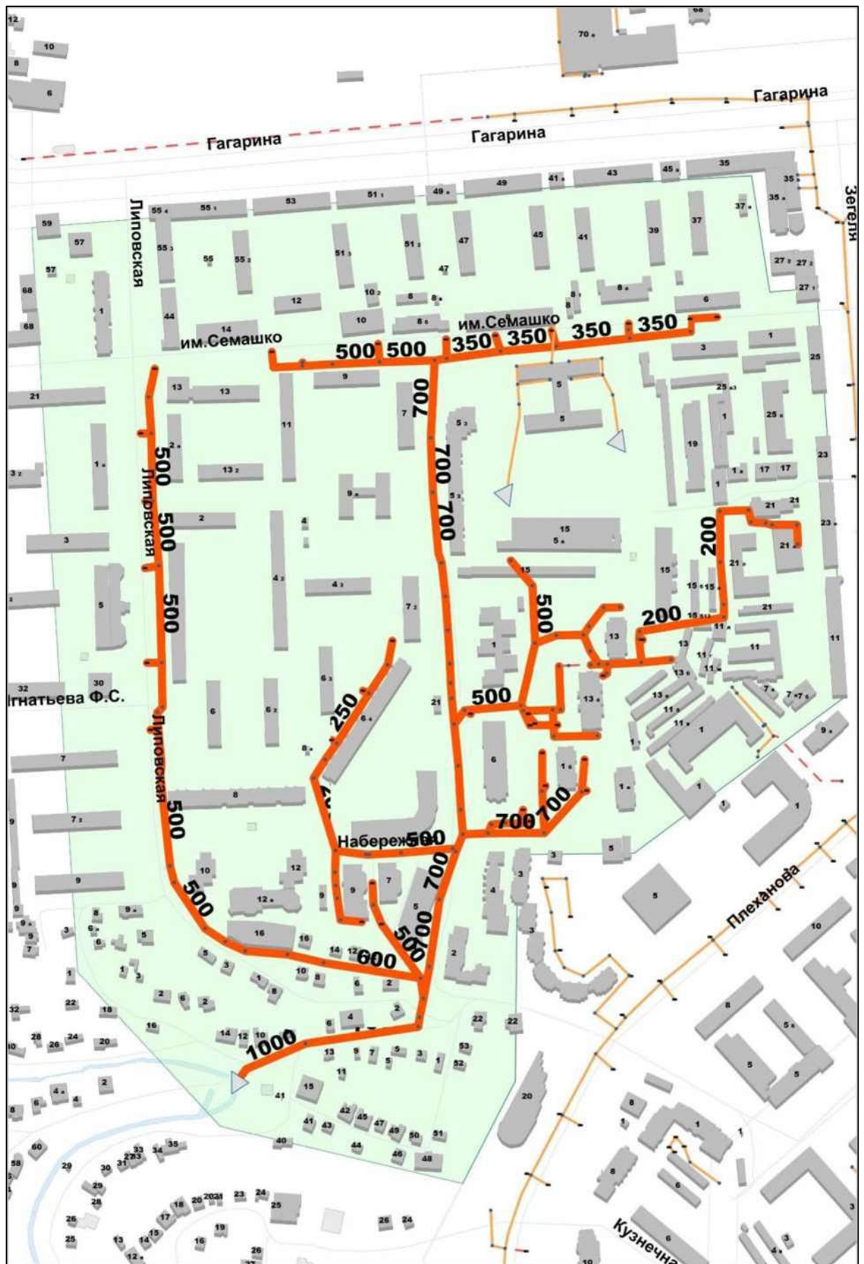
Рисунок 9 – Технологическая зона № 8
