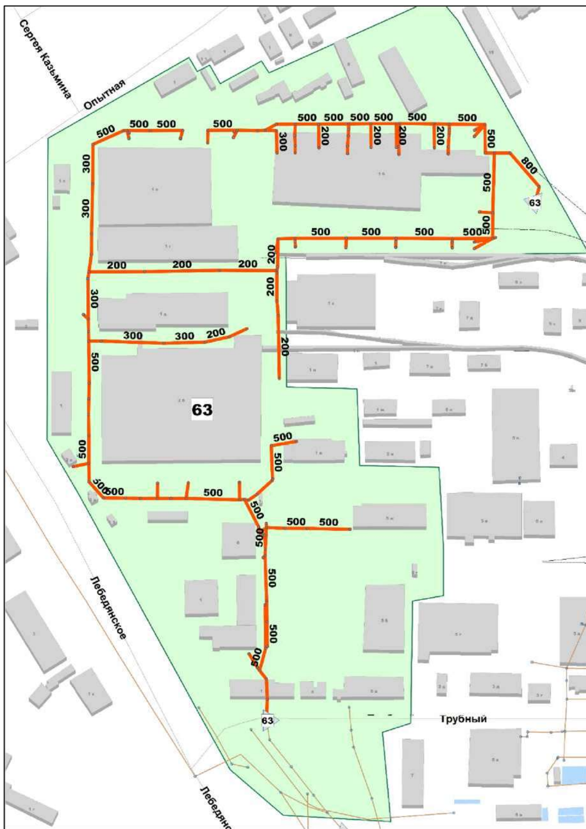
Рисунок 62 – Технологическая зона № 63
