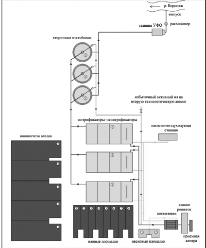
Рисунок 1.2.2. Технологическая схема очистки сточных вод на ЛОС ПАО «ЛПМК»
