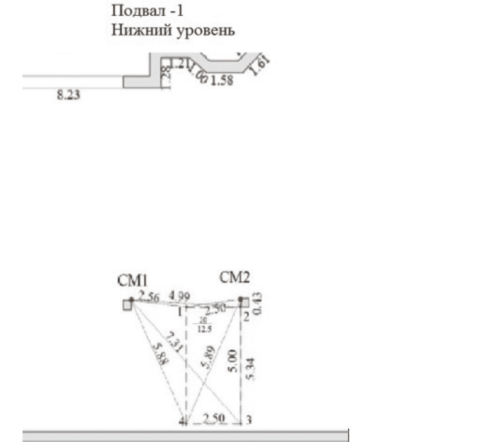
Фрагмент графической части проекта технического плана образуемого машино-места
